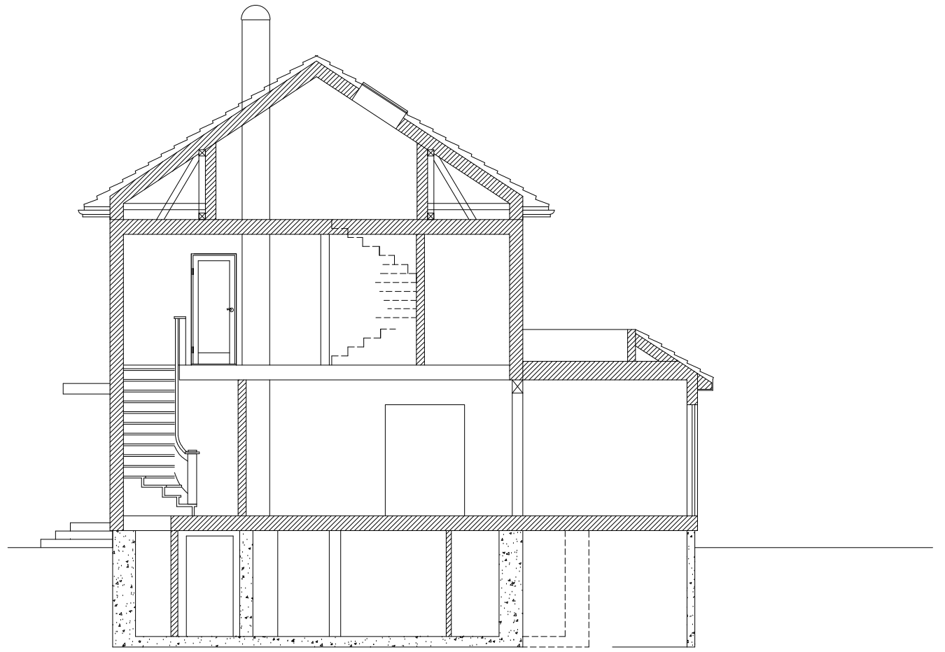
SNITT B-B
