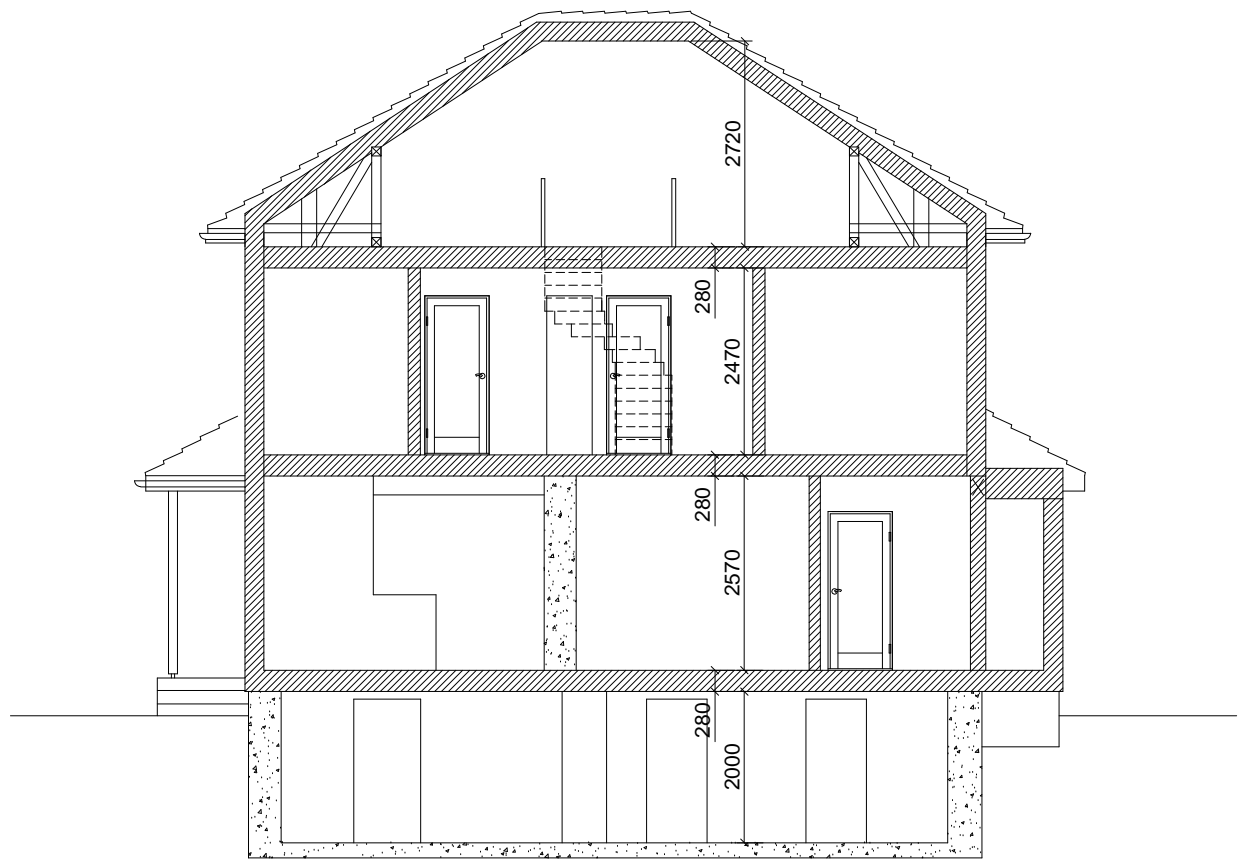
SNITT A-A
