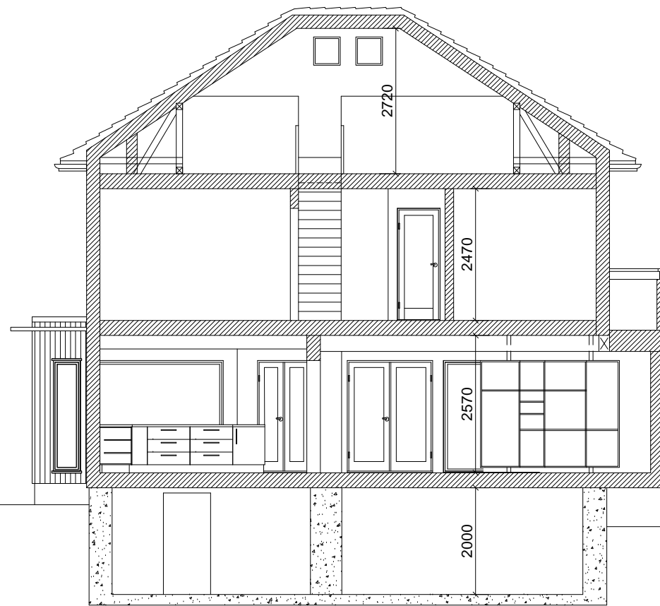
SNITT A-A
